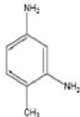
2,4-diaminotoluene
