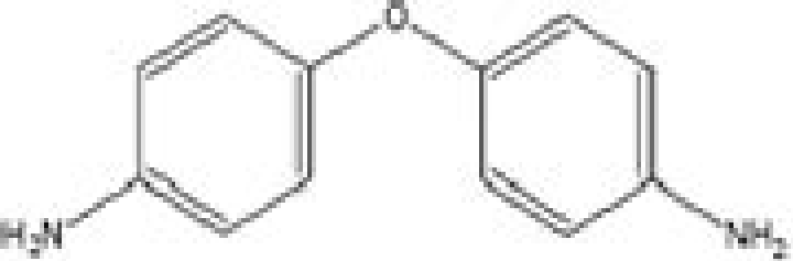
4,4'-oxydianiline
