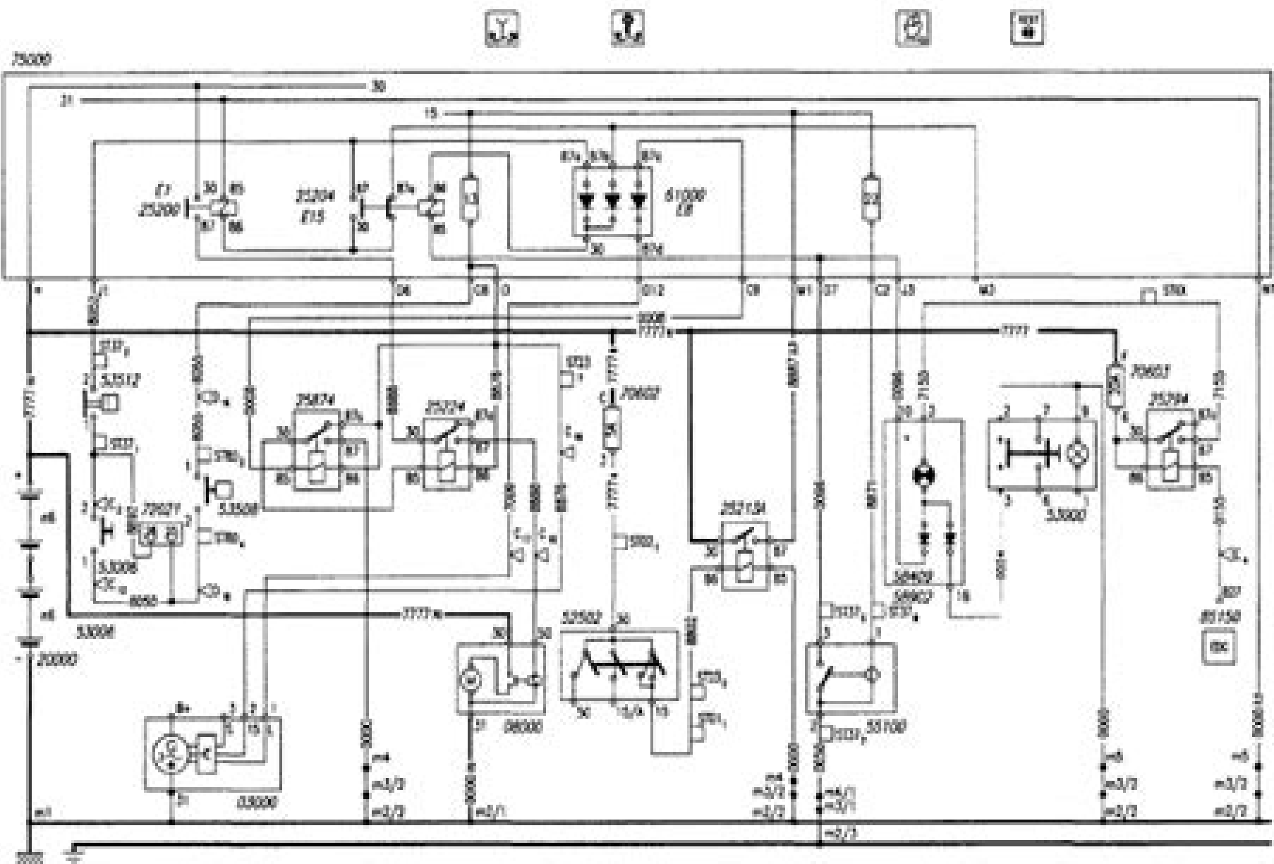
Схема № 2: Пуск двигателя из моторного отсека
