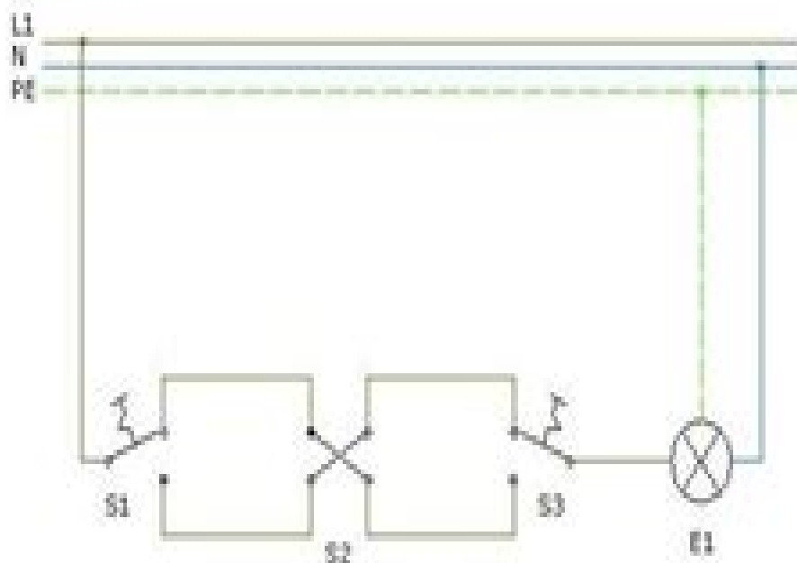
INSTALACIÓN DE UN PUNTO DE LUZ CONMUTADO DESDE TRES LUGARES
