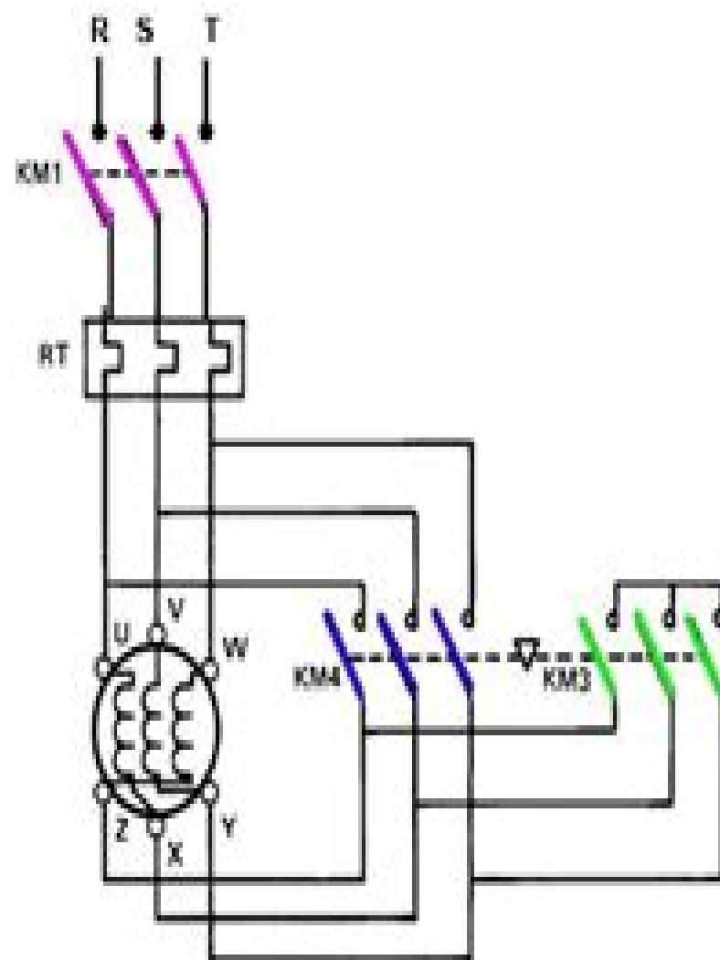
ARRANQUE DE UN MOTOR ESTRELLA-TRIÁNGULO ESQUEMA DE POTENCIA
