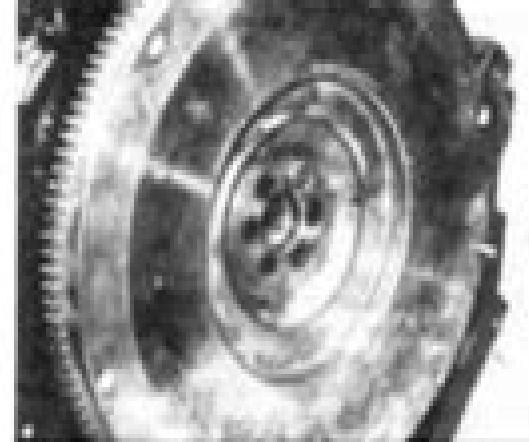
70.21. Снимите маховик.
