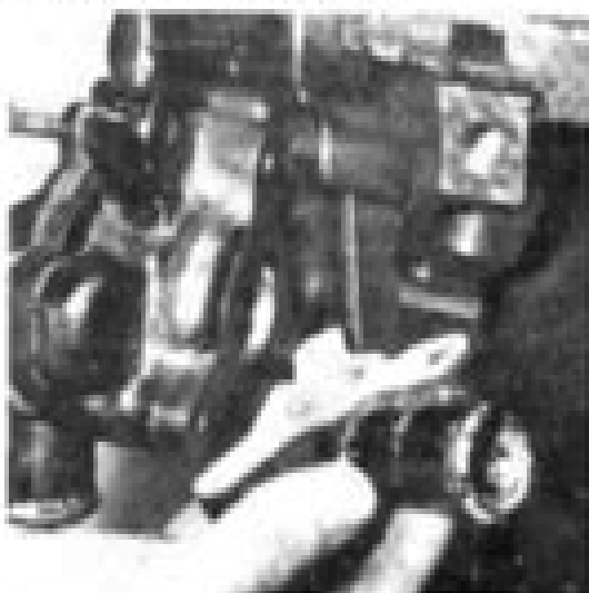
70.27. Снимите заднюю петлю водной магистрали.
