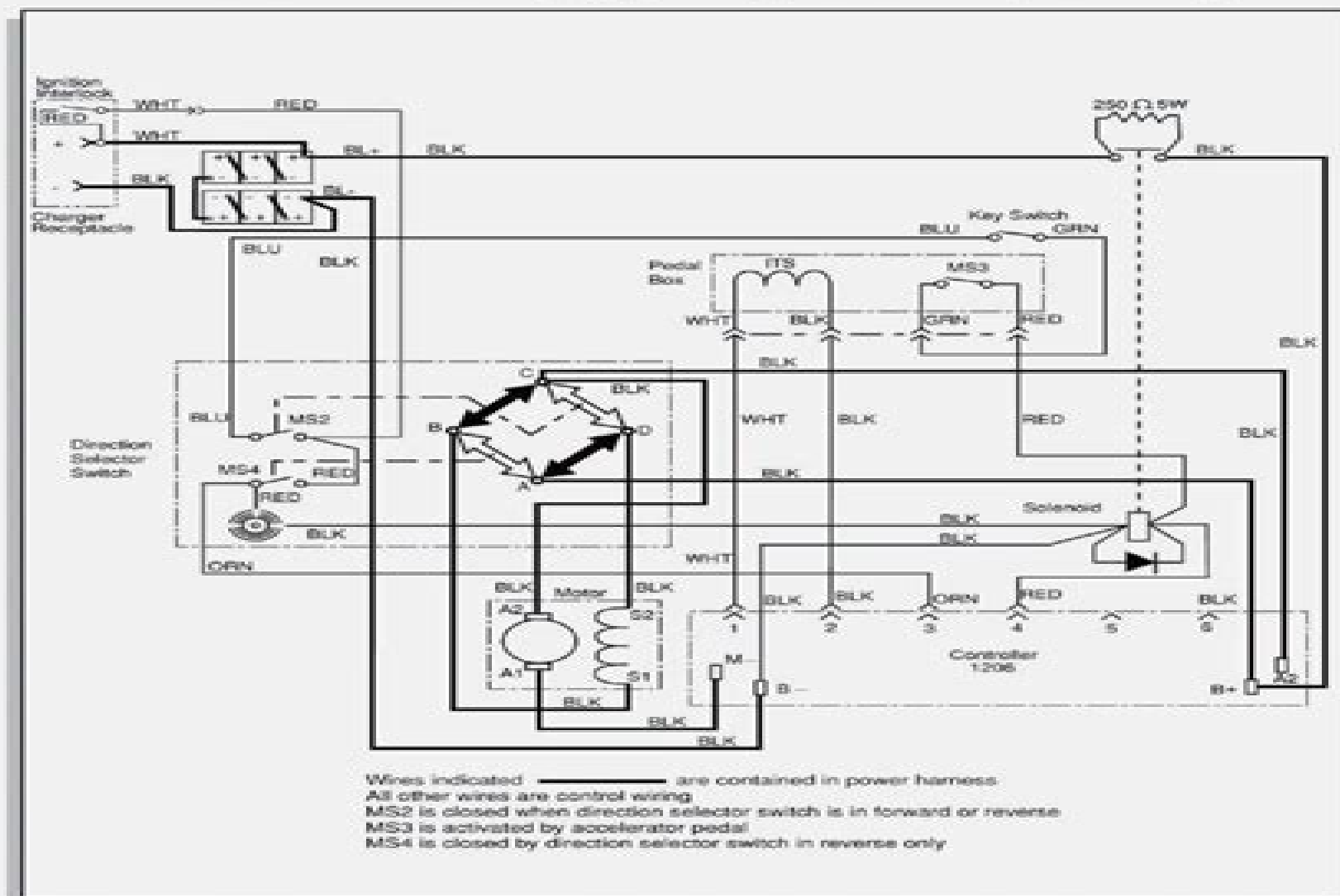
Fig. 19 Wiring Diagram
