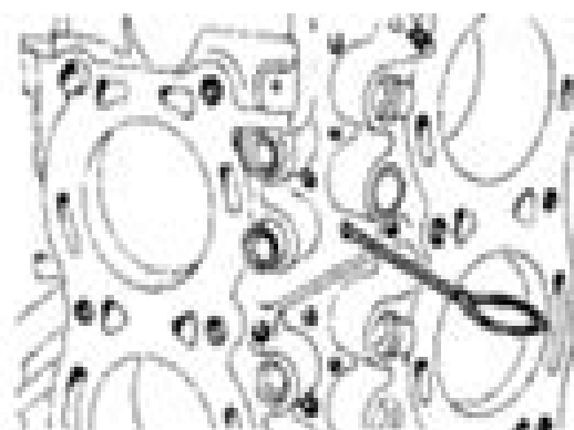
Рис. 1.23. Использование проволоки для снятия толкателей.
