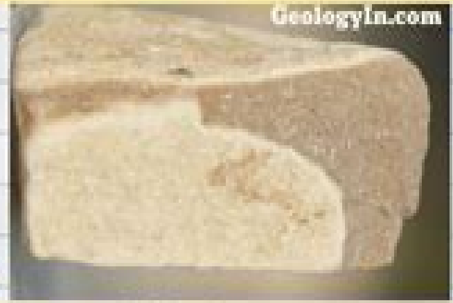
Mudstone
